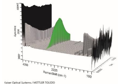
Ramanspektrum mit gemessenem Methanpeak (grün) während der CO 2 -Methanisierung des Eisenkatalysators
