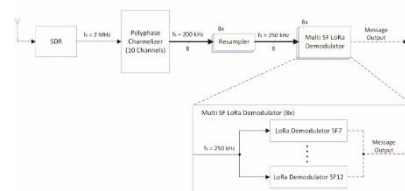
Systemübersicht des LoRa-Sniffers
